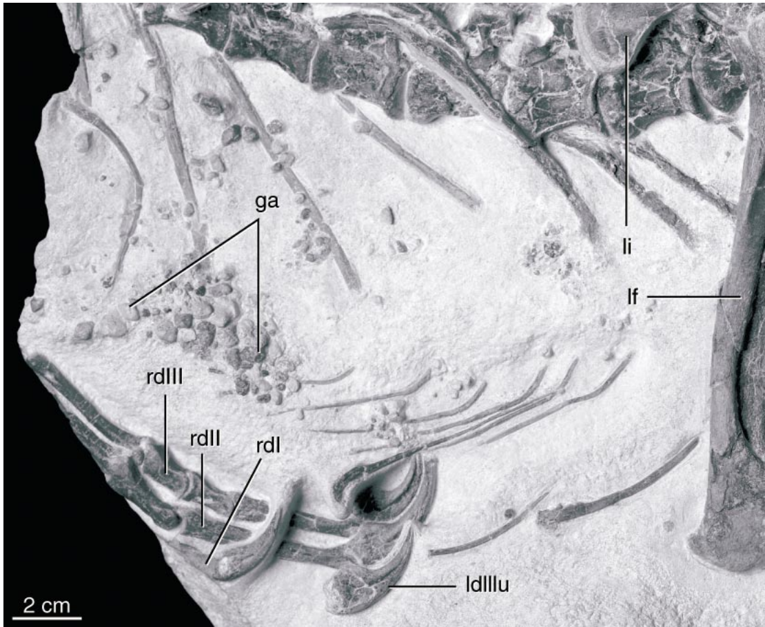
Fig. 9. Gastroliths of Shenzhousaurus orientalis . ga, gastroliths; ldIIIu, left digit 3 ungual; lf, left femur; li, left ilium; rdI, right digit 1, rdII, right digit 2; rdIII, right digit 3.
